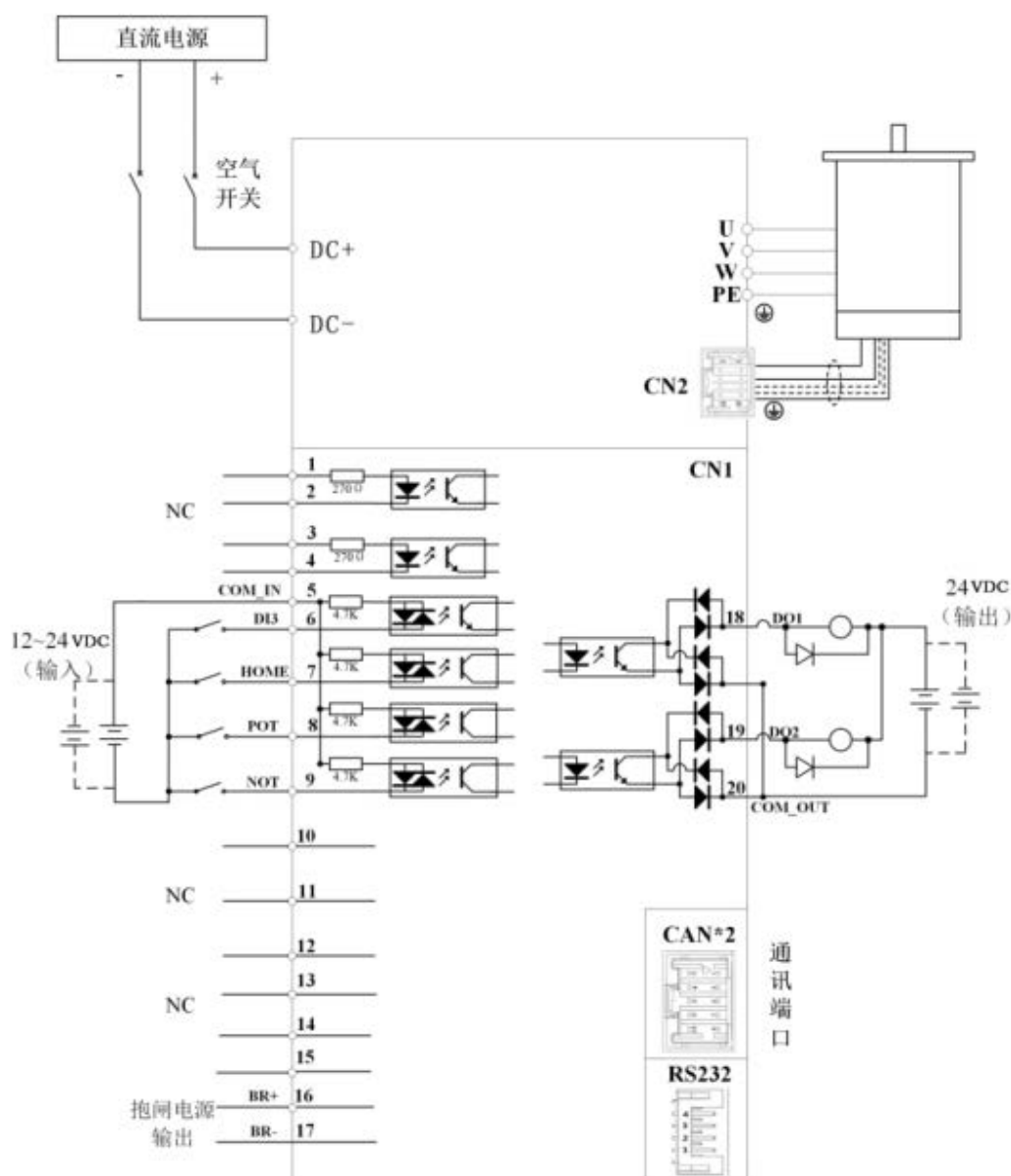
图 3.1 标准接线
