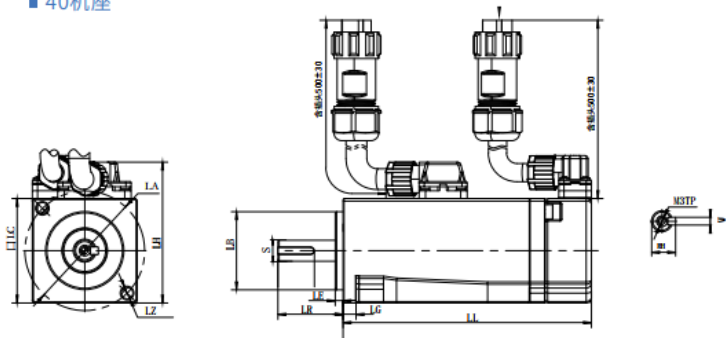
■ LVM系列电机机械尺寸 ■ 40机座
