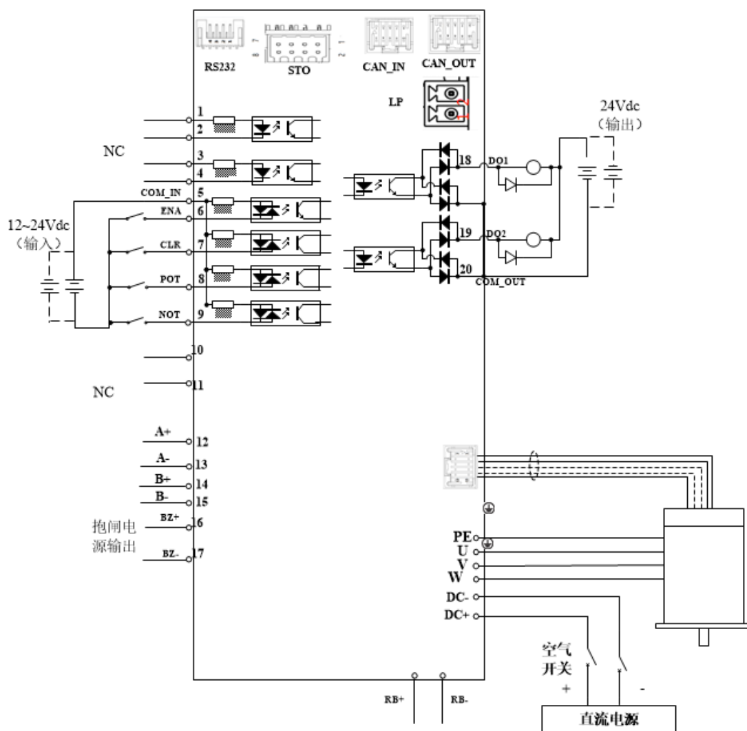
图 3.2 标准接线
