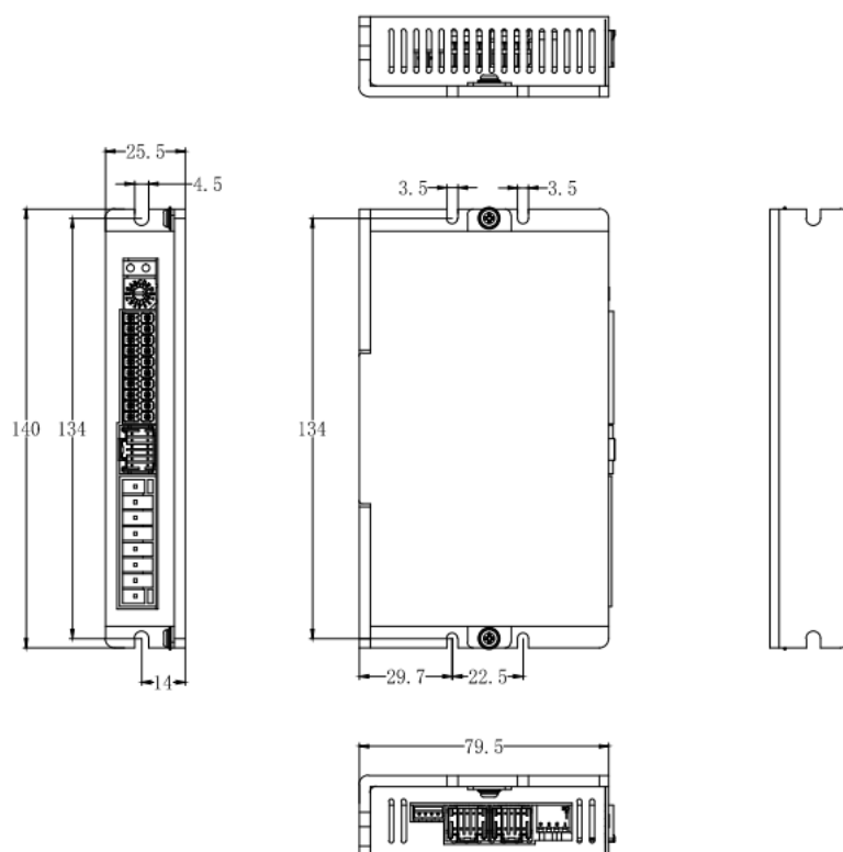
图 2.2 LD2-7010/07/05 驱动器底板安装方法
