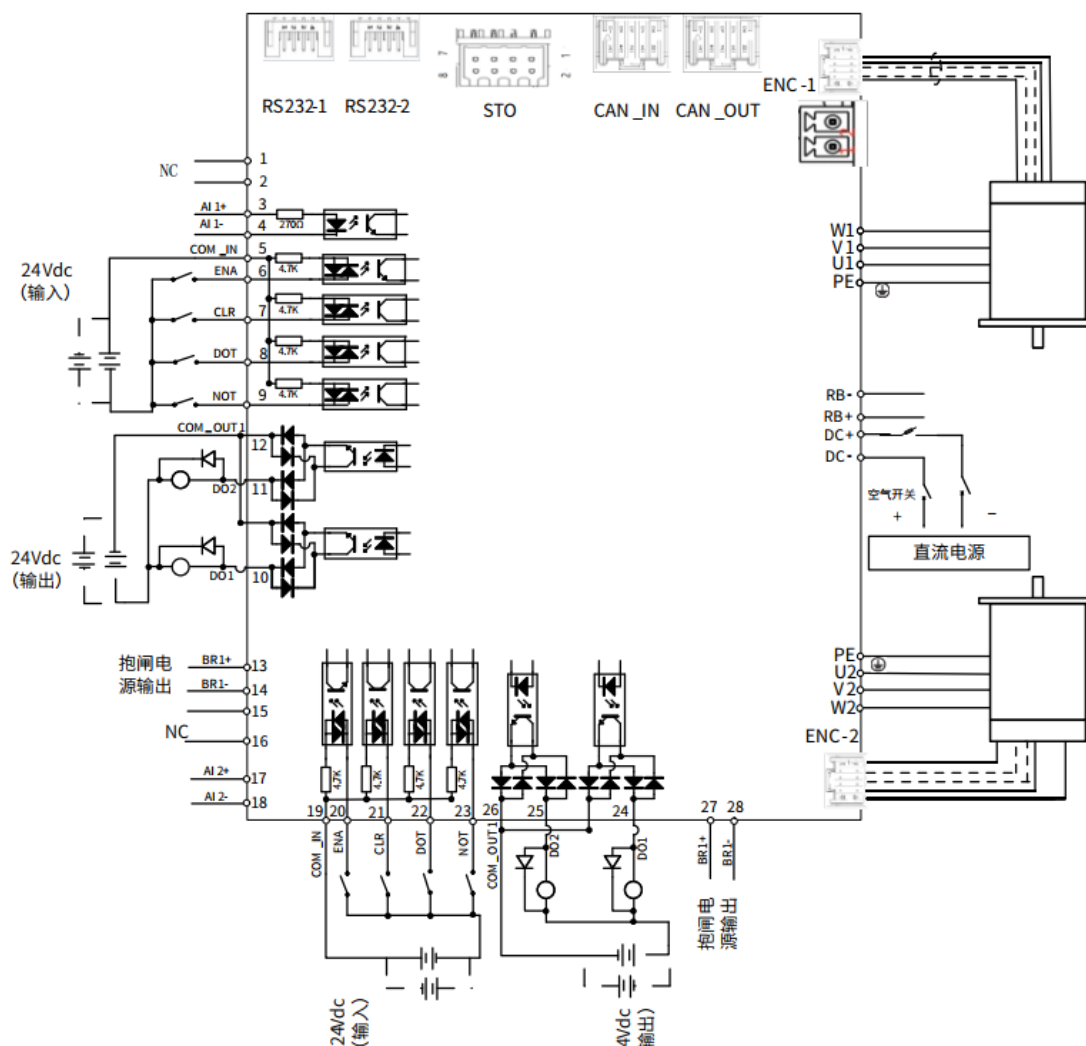
图 3.3 标准接线
