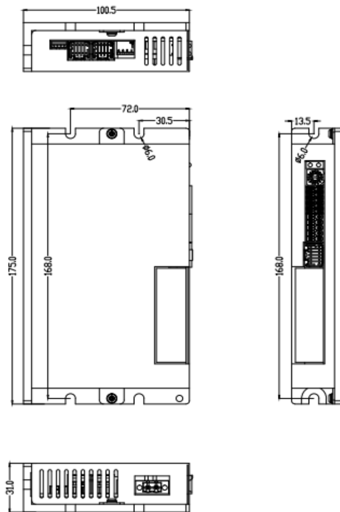
图 2.1 LD2-7030/20/15 驱动器底板安装方法
