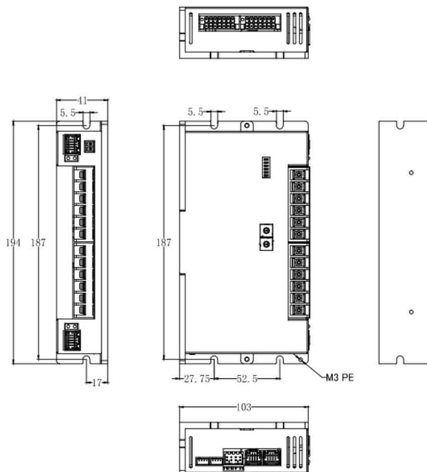
图 2.4 2LD2-系列（2LD2-7030,2LD2-7020,2LD2-7015）驱动器底板安装方法
