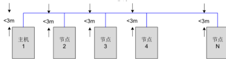
图 4 多台 CAN 驱动器组网结构图
