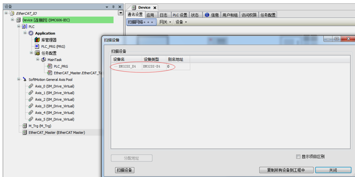
图 6.12 扫描网络
