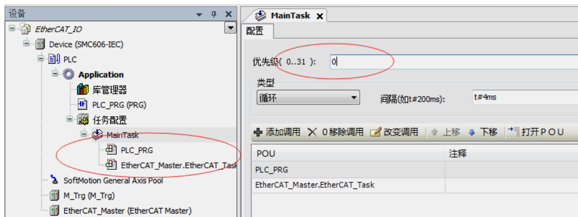
图 6.3 配置任务
