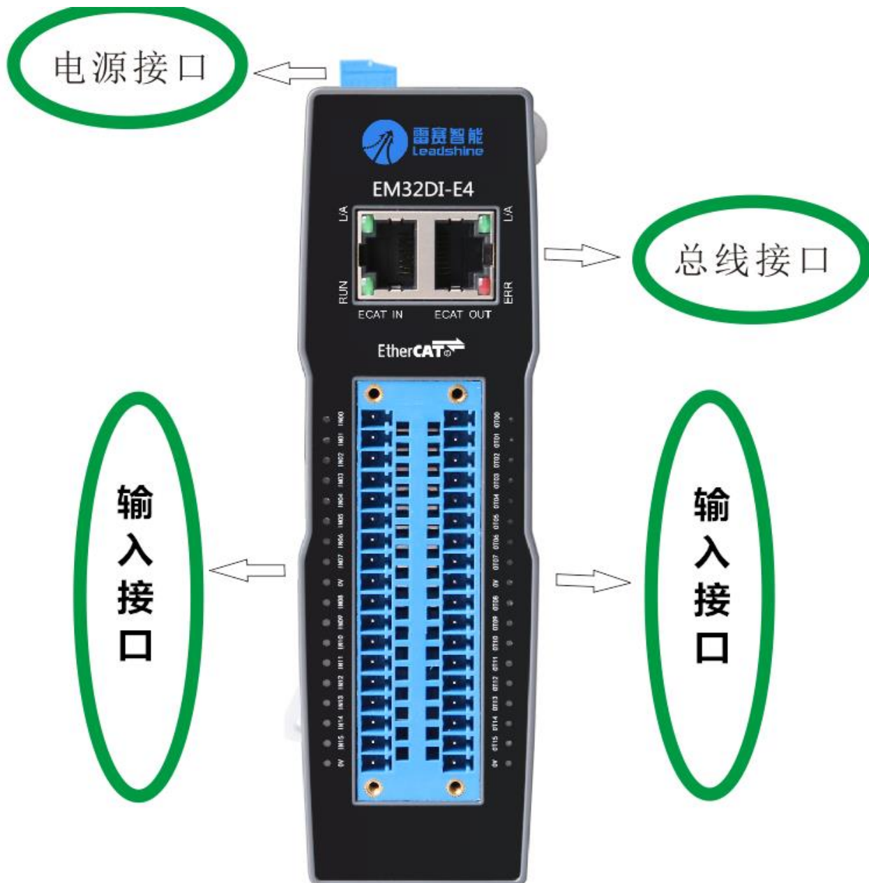
图 2.2 EM32DI-E4 硬件接口分布图
