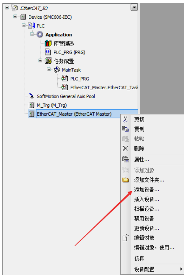
图 6.8 添加设备
