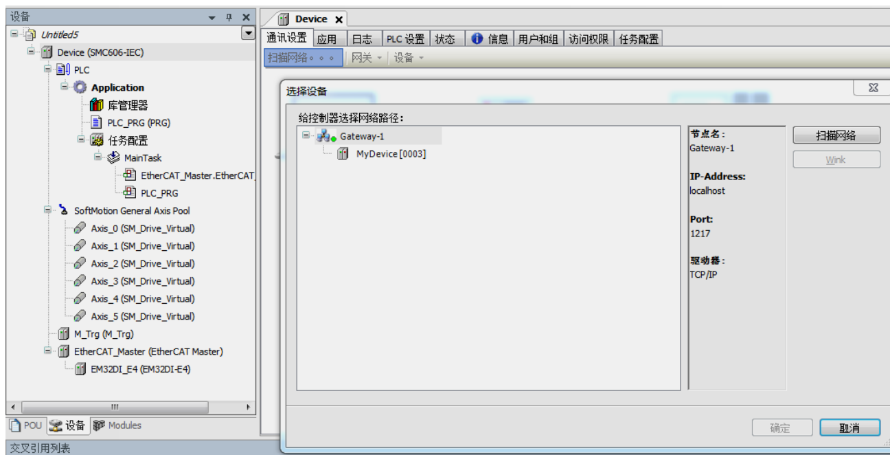
图 6.10 扫描网络
