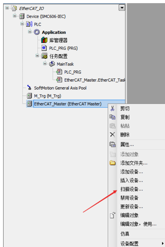
图 6.11 扫描设备
