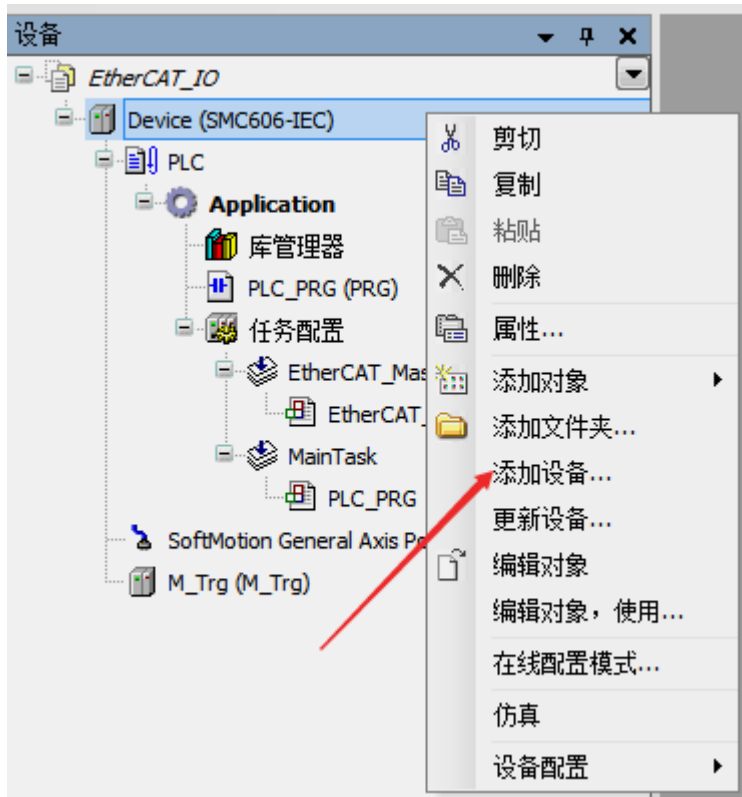
图 6.1 添加设备
