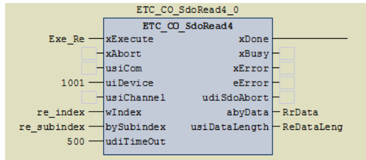
图 5.20 SDO 读取功能块
