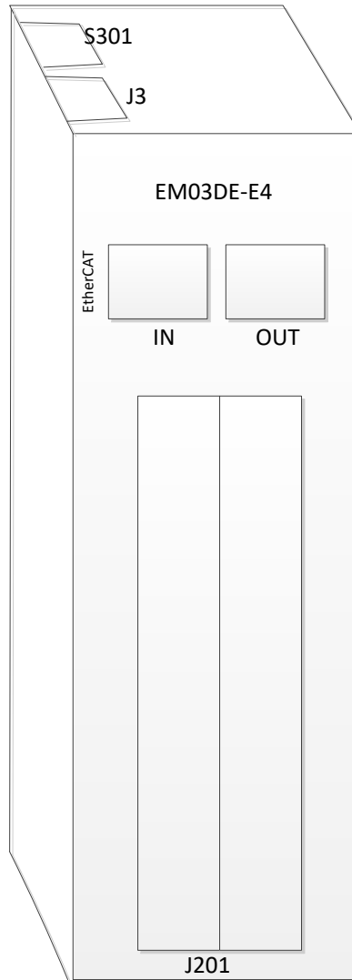
图 2.2 EM03DE-E4 模块硬件接口分布图
