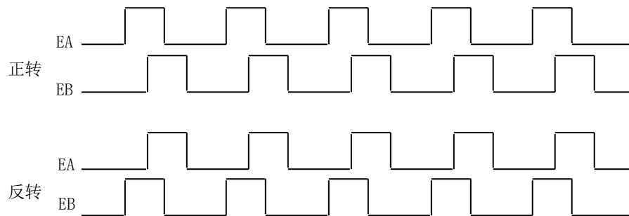
图 2.4 A/B 相正交信号
