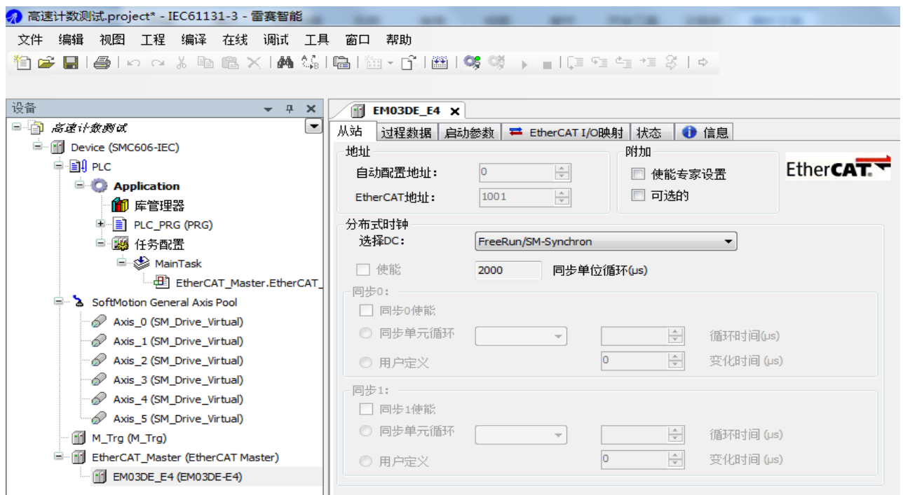
图 5.3 设备树
