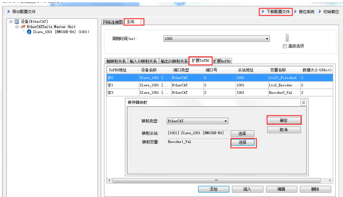
图 5.70 变量映射
