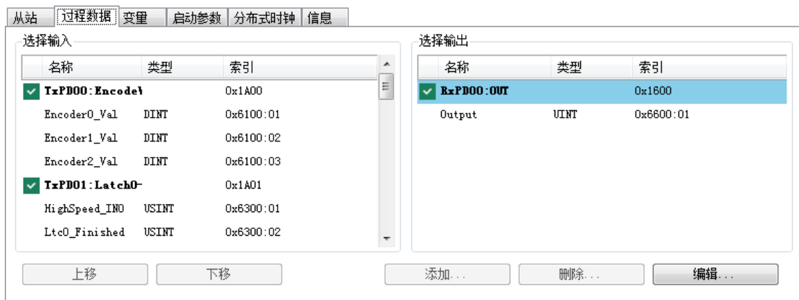
图 5.39 过程数据
