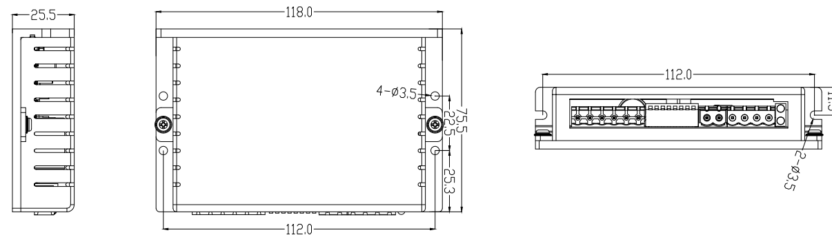
DM1-442C、DM1-542C、DM1-556C安装尺寸图
