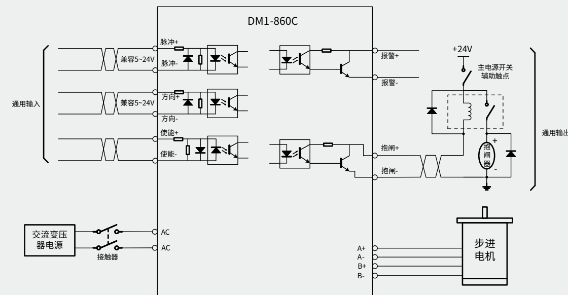
DM1-860C接线图
