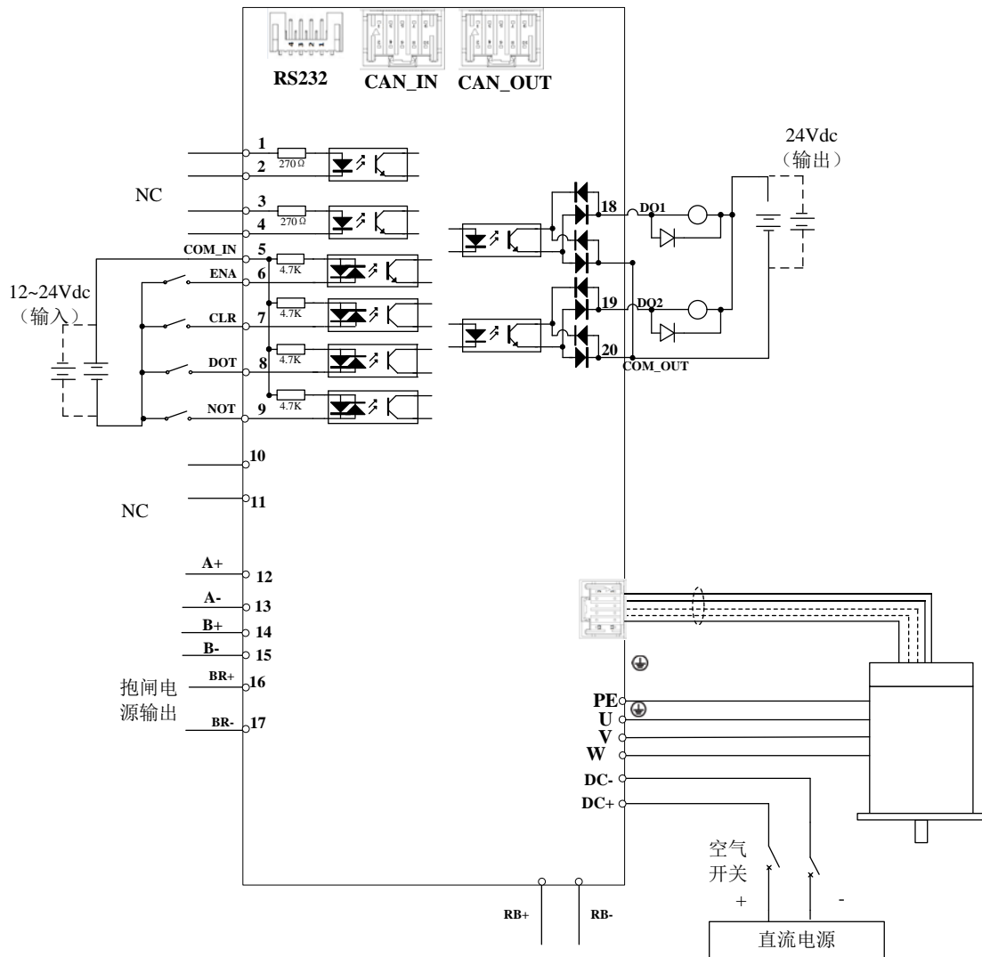
图 3-1 标准接线
