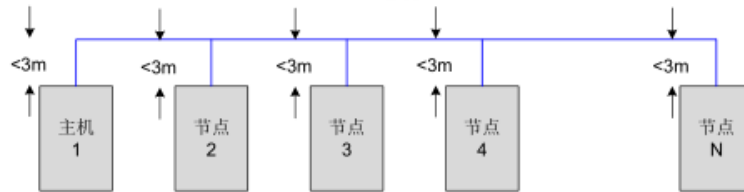
图 4 多台 CAN 驱动器组网结构图
