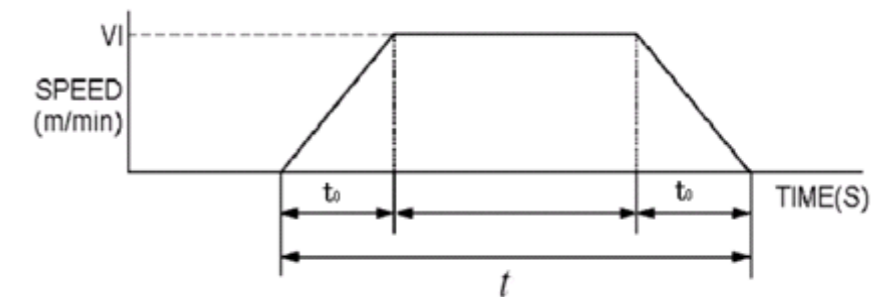
图3: 运行曲线
