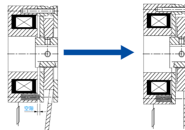
断电释放
