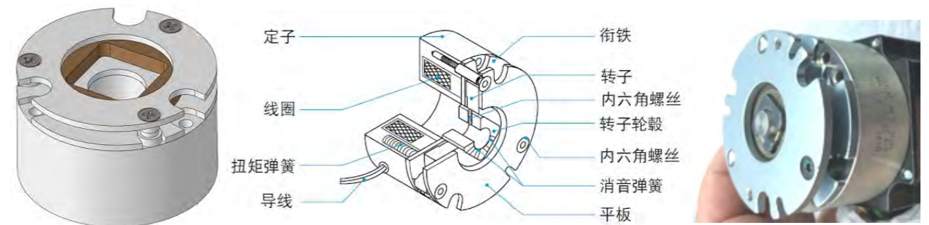
结构3D图
