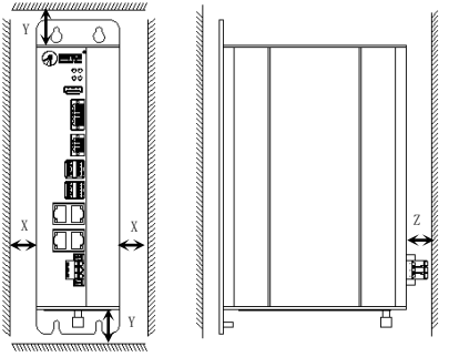
背面挂耳支架安装
