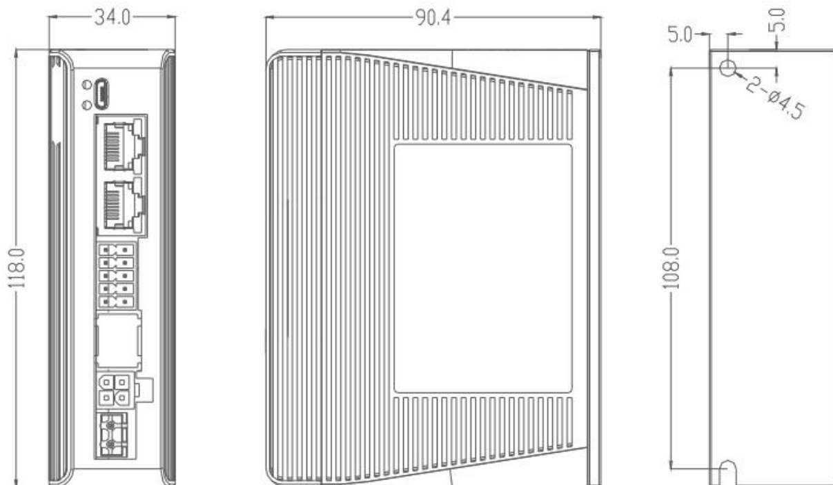
图 2-1 DM3C-522/556/870 安装尺寸图(单位: mm)
