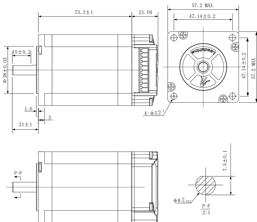
图 1 安装尺寸图
