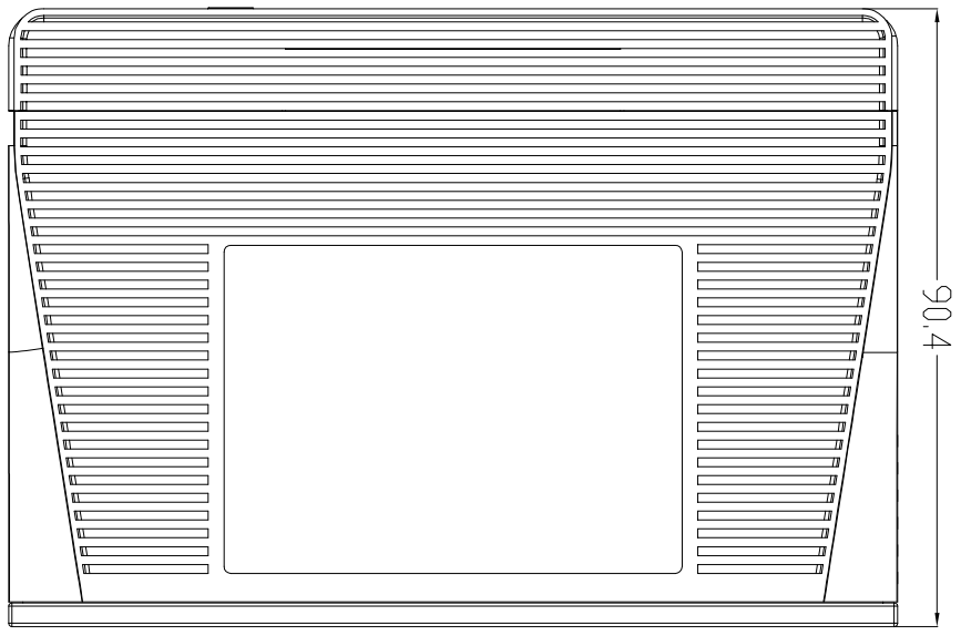
主视图
