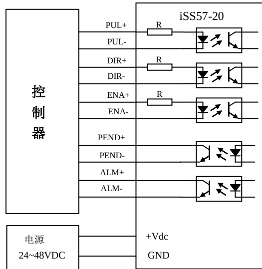
图 6 典型接线图
